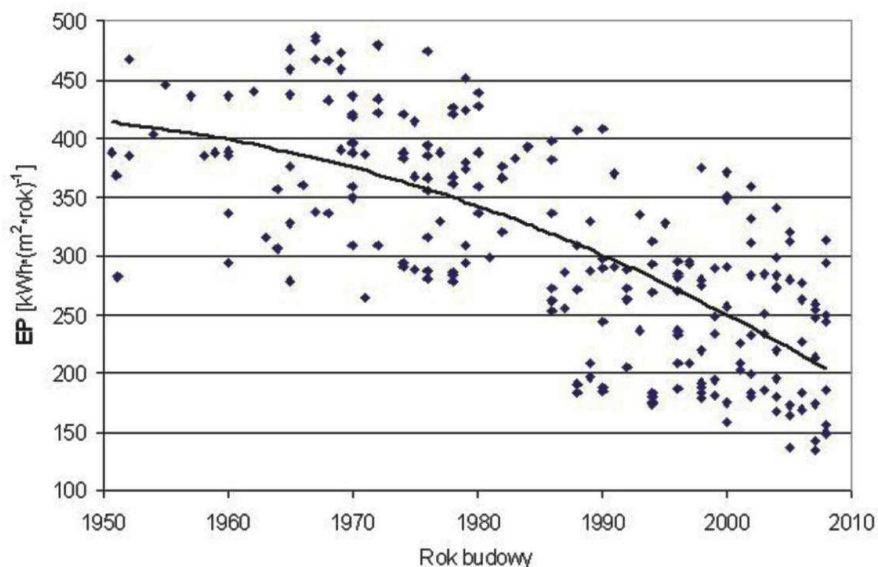
Rys. 2. Wielkość wskaźnika rocznego zapotrzebowania na energię pierwotną EP zależnie od roku budowy budynku.
